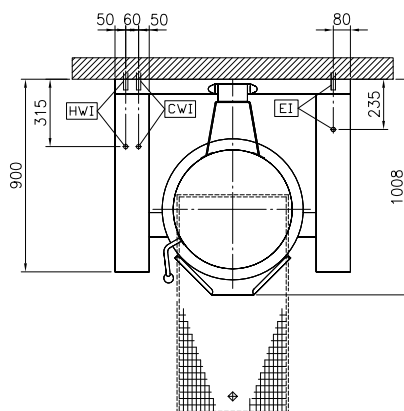
Boven aanzicht
